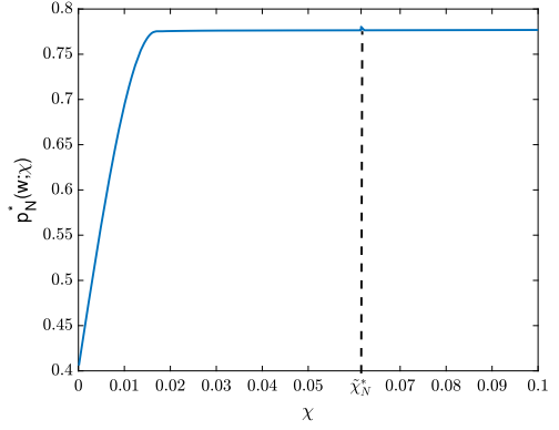
(b) p_N^*(\chi)
