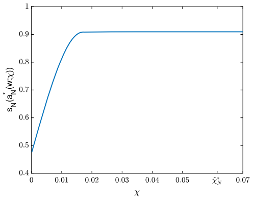
(d) s_N(\chi)
